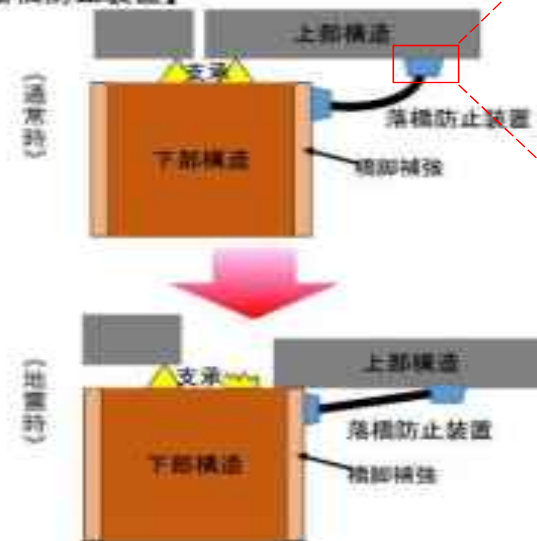
【落橋防止装置】
